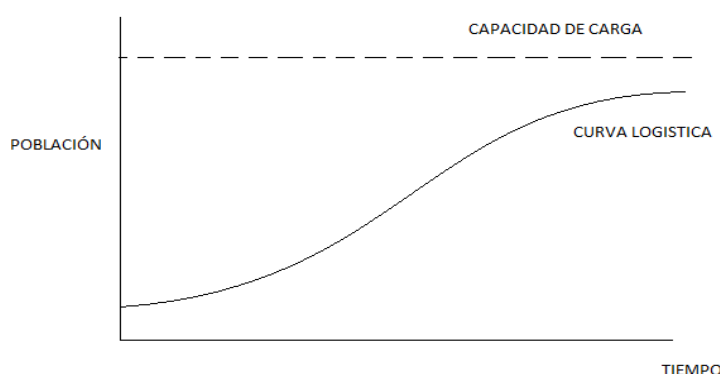
Gráfico 2 Función logística
