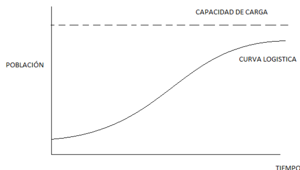
Gráfico 2 Función logística
